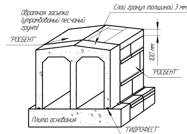
Рис. 21 Укладка матов «Росбент» для гидроизоляции тоннелей
