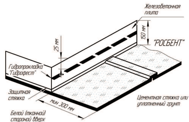
Рис. 3 «Росбент» укладывается на подготовку – цементную стяжку или уплотненный грунт и требует установки плиты толщиной не менее 150 мм.
