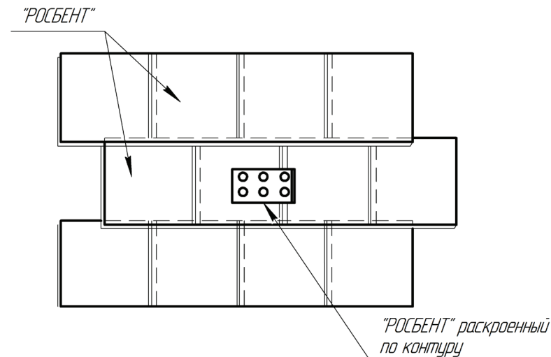
Рис. 11 Раскрой и укладка «Росбента» в местах конструкций, проходящих через стену
