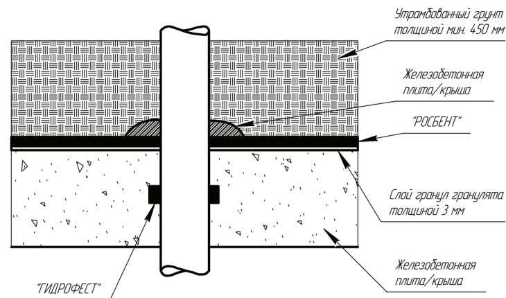
Рис. 8 Прохождение инженерных коммуникаций или строительных элементов через покрытую землей крышу.
